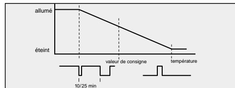
Schéma 1: Courbe caractéristique du rapport entre les impulsions et les pauses en fonction de la température
