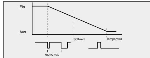
Bild 1: Verlauf der relativen Einschaltdauer (Tastverhältnis) in Abhängigkeit von der Temperatur
