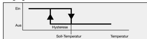
Bild 2: 2-Punkt-Regelung
